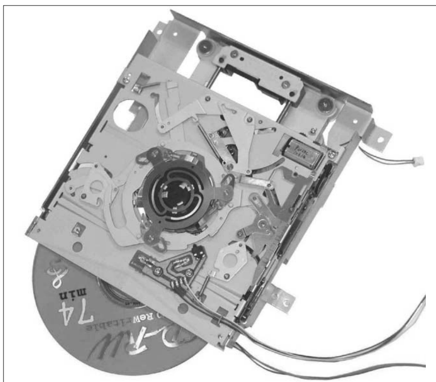
Рис. 1. Внешний вид узла проигрывателя
