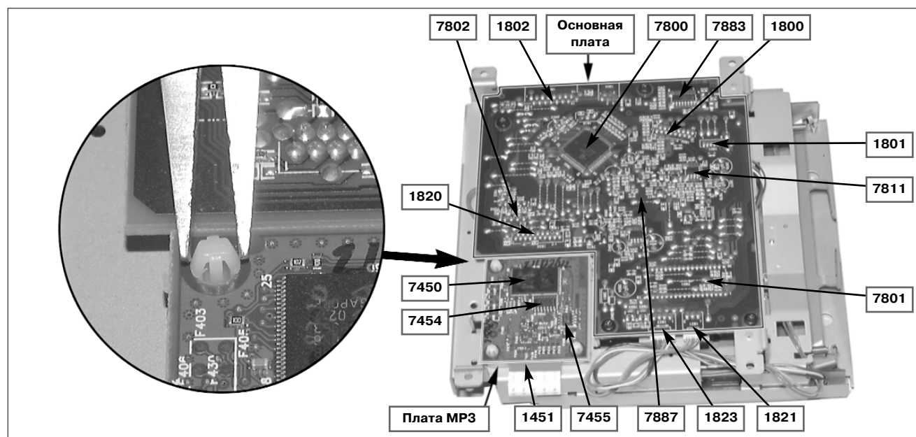
Рис. 2. Внешний вид электронных плат узла проигрывателя
