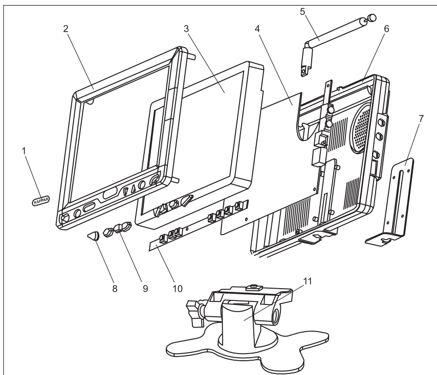
Рис. 1. Конструктивные элементы телевизоров: 1 — логотип; 2 — передняя панель; 3 — ЖК панель; 4 — главная плата; 5 — антенна; 6 — задняя крышка; 7 — металлический кронштейн; 8 — окно фотоприемника; 9 — пластмассовые кнопки; 10 — плата с кнопками; 11 — подставка
